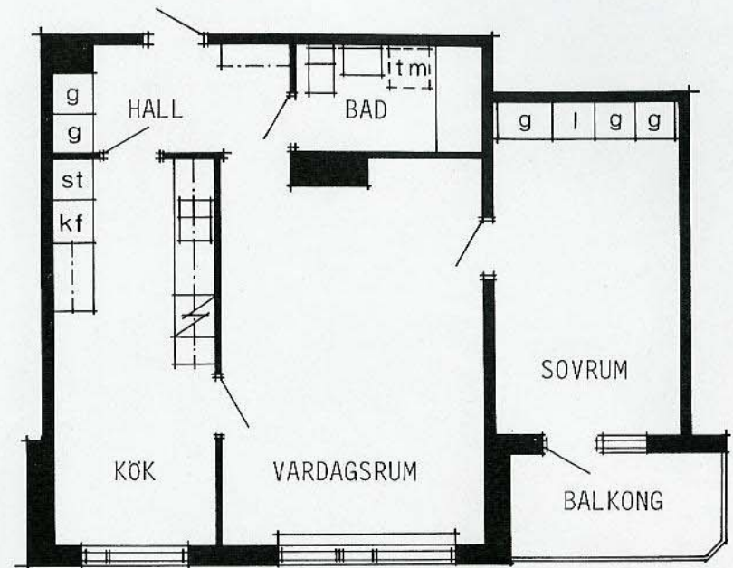
Typ 2 2 R o K 60,3 m 2 Totalt 10 st: Nr 5, 8, 11, 14, 17, 45, 48, 51, 54, 57
